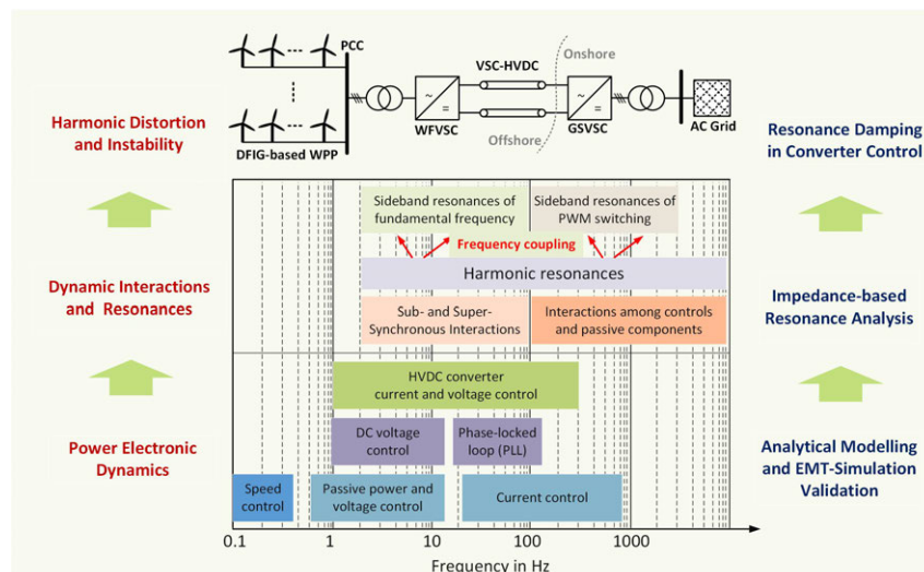
Abbildung 3.28: Schwingungen in OWF mit HGÜ-Anschluss: Modellierung, Analyse und aktive Dämpfung
