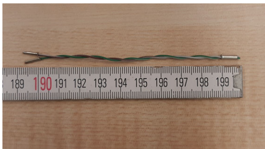
(a) 10 cm lange leerlaufende Zweidrahtleitung
