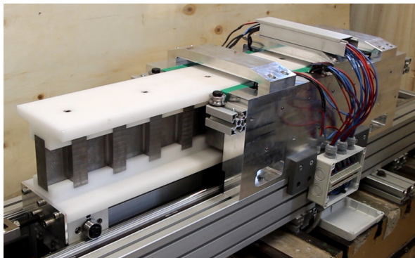
(a) Linearanordnung
