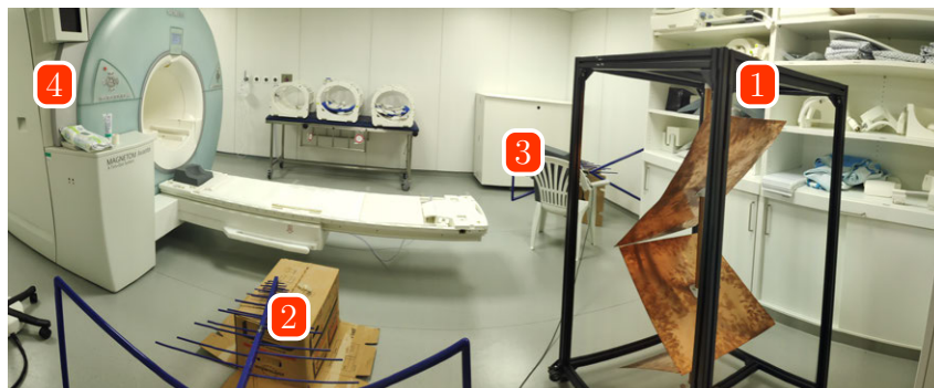
Abbildung 3.32: Messaufbau der Gütemessung: 1 Rührer; 2 Empfangsantenne; 3 Sendeanenne; 4 MRT Magnetom Avanto
